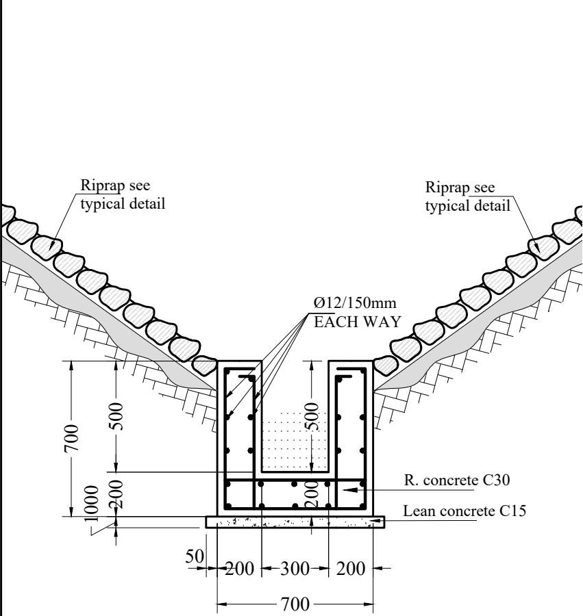
SECTION G-G 1:20
