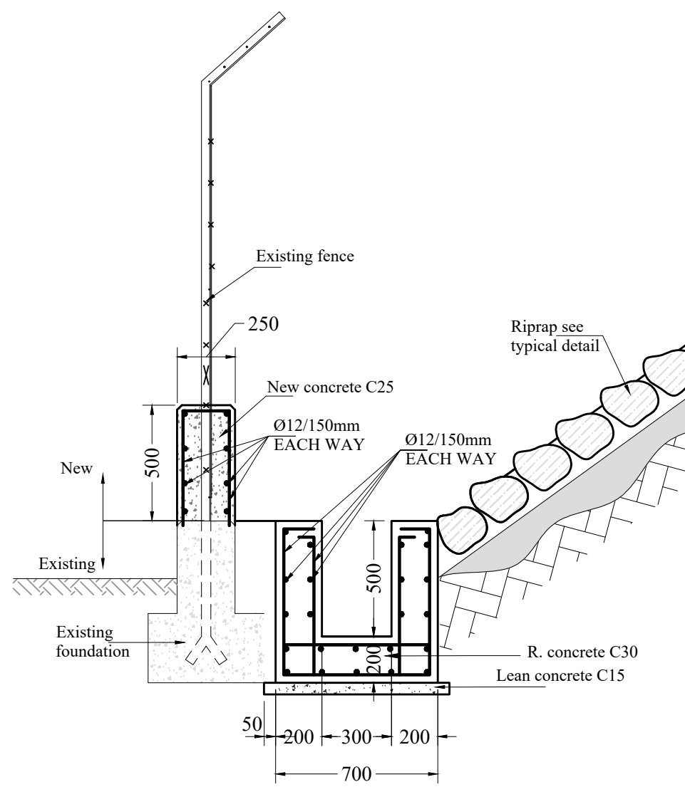
SECTION E-E 1:20
