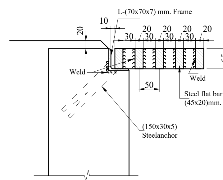
DETAIL-1 1:5
