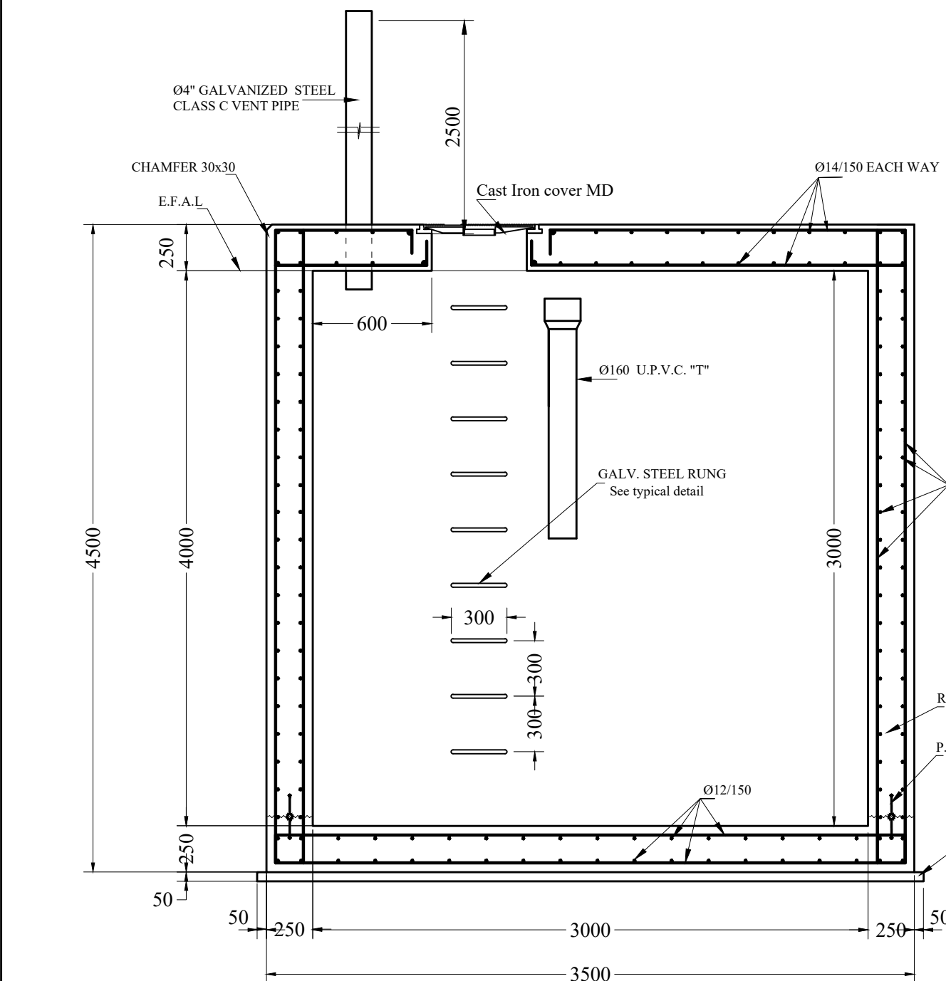
SECTION D-D 1:20
